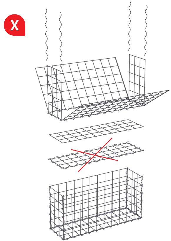
EIN BEISPIEL FÜR DIE MONTAGE VON ÜBEREINANDER GESTAPELTEN GABIONENKÖRBEN
