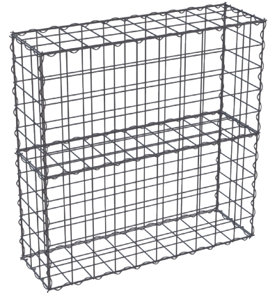
EIN BEISPIEL FÜR DIE MONTAGE VON ÜBEREINANDER GESTAPELTEN GABIONENKÖRBEN
